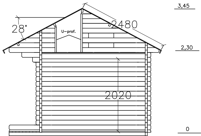
LEIKKAUS A - A
